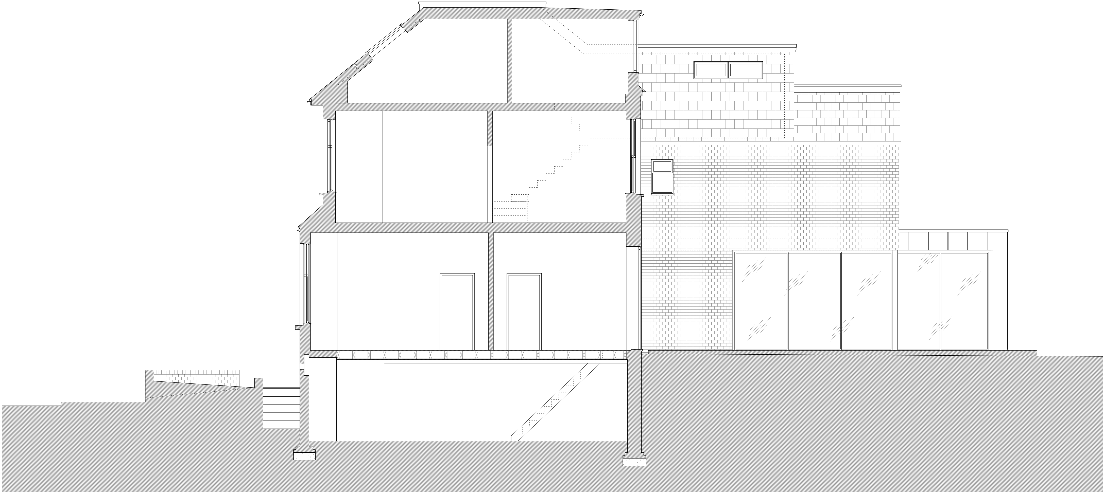
1 Existing Section A Scale: 1:50 @ A1 & 1:100 @ A3
