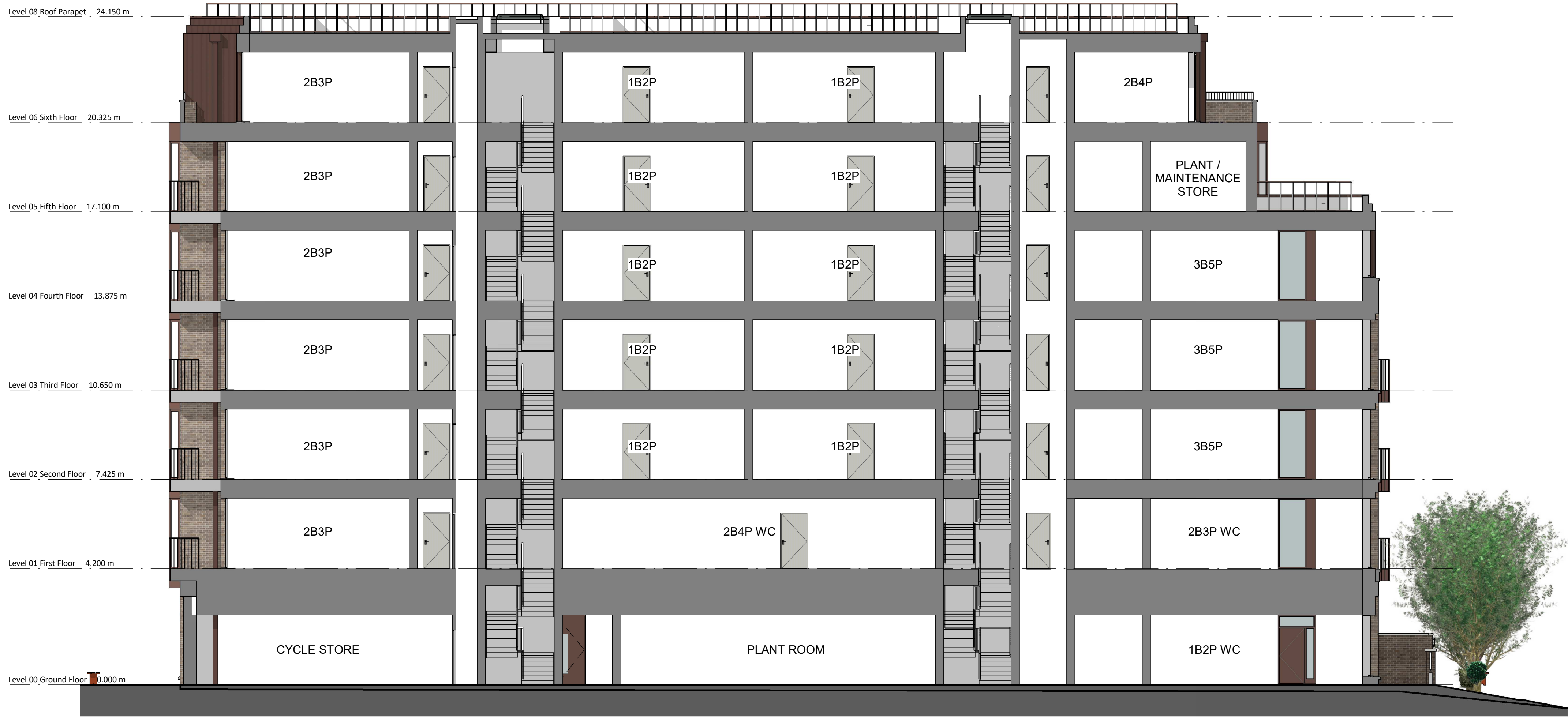
Section A-A 1 : 100
